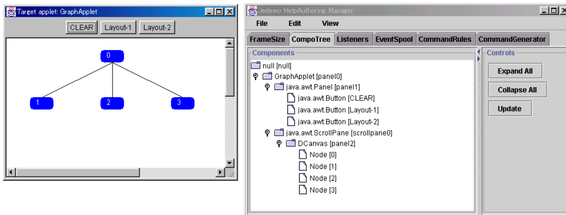
図 2 JedemoAuthor : 対象アプレットと含まれる部品の階層構造 Fig. 2 JedemoAuthor: The target applet and its component structure.
