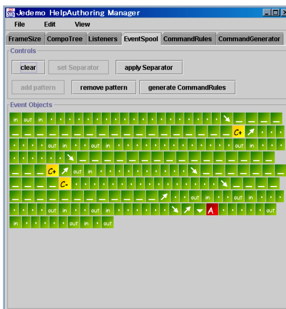
図 3 JedemoAuthor : スプールに保存されたイベントオブジェクト Fig. 3 JedemoAuthor: Recorded event objects.
